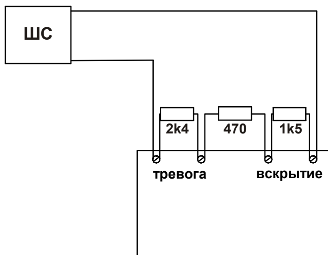
Рис. 8 Пример подключения в шлейф извещателя с отдельными клеммами датчика вскрытия и сигнала тревоги.
