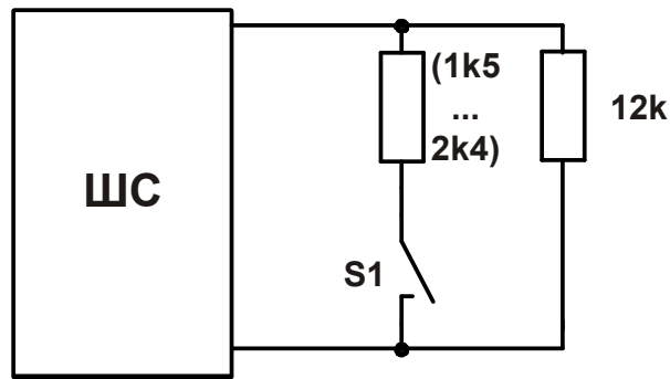
Рис. Схема 4 Параллельное подключение 1-го извещателя с НР контактами.
