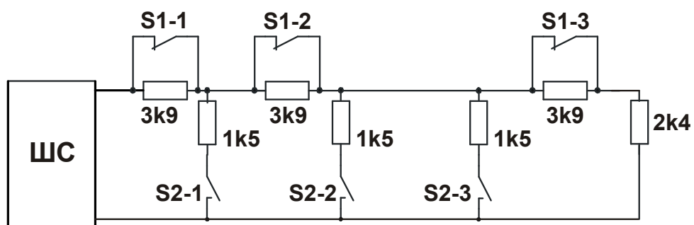
Рис. Схема 7. Параллельно-последовательное подключение и НЗ и НР извеща
