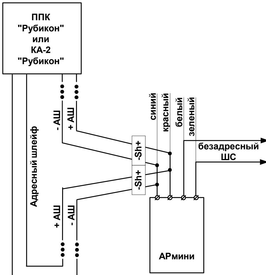
Рис. 2 Подключение АРмини с одним ШС
