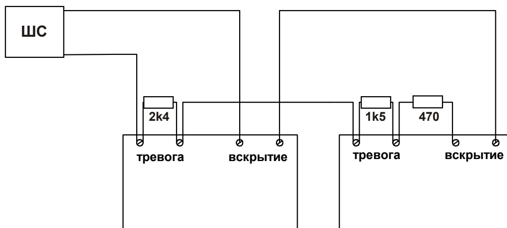
Рис. 9 Пример подключения в шлейф двух извещателей с отдельными клеммами датчика вскрытия и сигнала тревоги.
