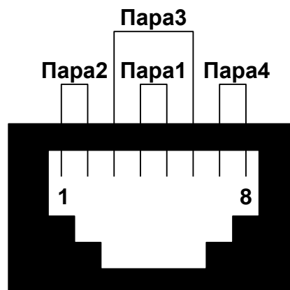
Рис. 6. Разводка RJ-45.
