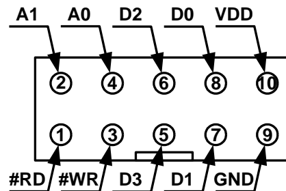
Рис. 5. Назначение контактов разъема ХТ1.
