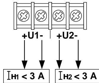
Рис. 4 Схема подключения нагрузки ( I_{n1} < 3A ; I_{n2} < 3A )
