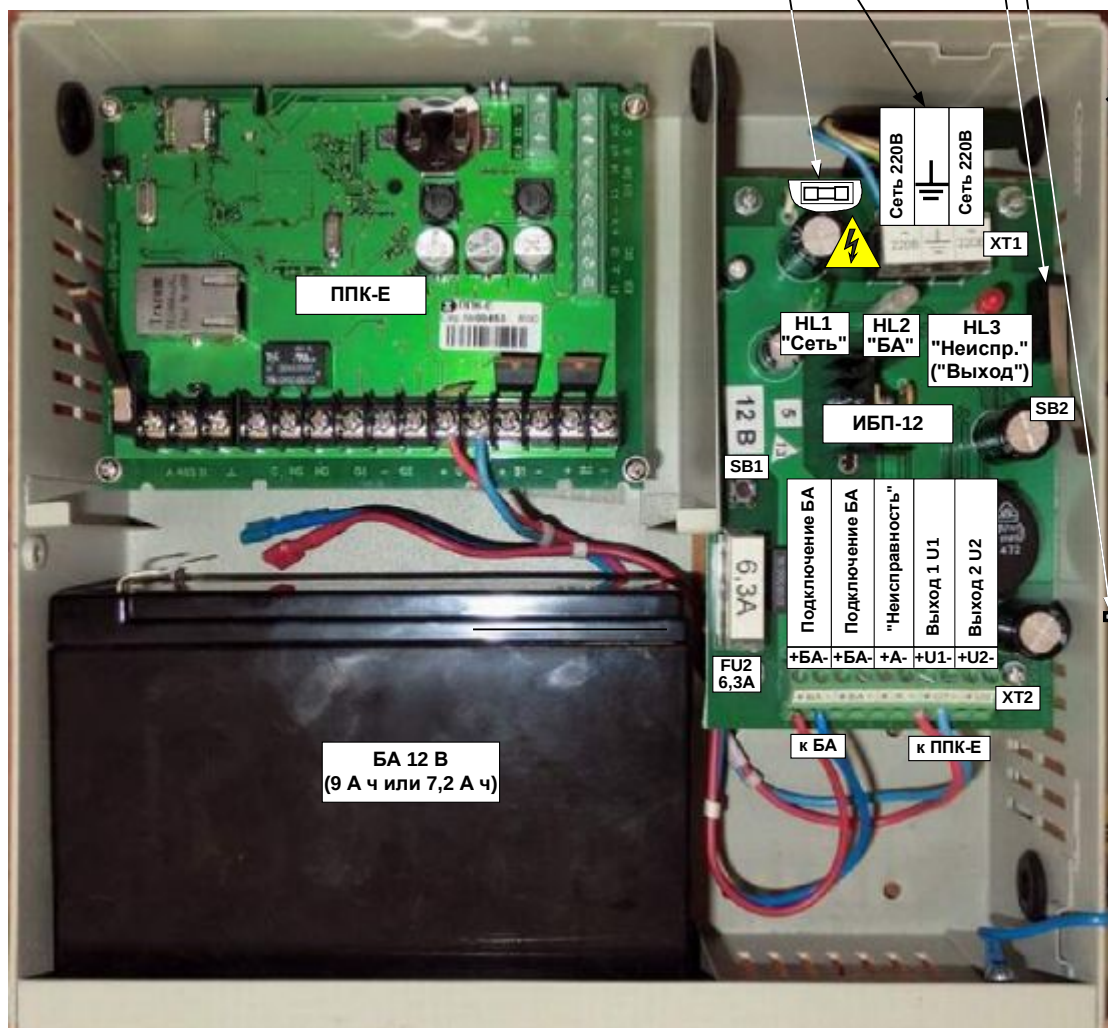
Рис. 11 Внешний вид ППК-Е (исп. 1)
