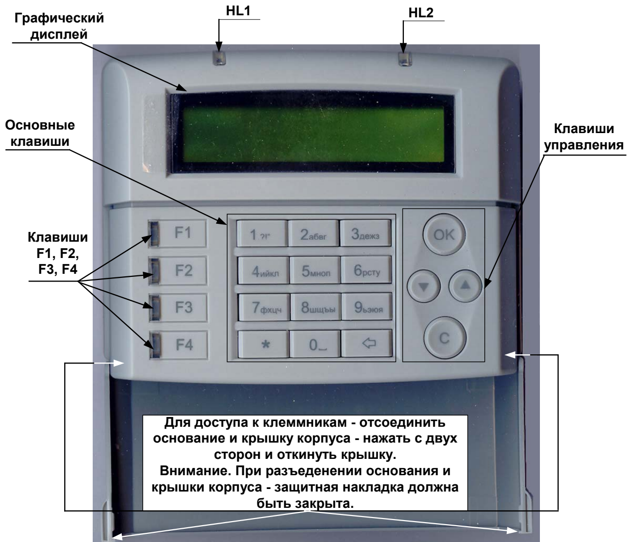
Рис. 2 Внешний вид ПУО (с откинутой накладкой)
