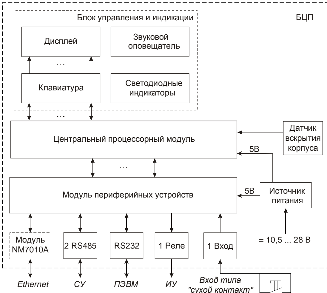
Рис. 6 Электрическая структурная схема БЦП Р-08 исп. 6
