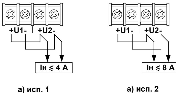
Рис. 6 Схема подключения нагрузки а) исп. 1 ( I_n \leq 4A ); б) исп. 2 ( I_n \leq 8A ).
