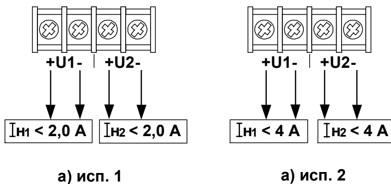
Рис. 5 Схема подключения нагрузки: а) исп. 1 ( I_{n1} < 2,0A ; I_{n2} < 2,0A ); б) исп. 2 ( I_{n1} < 4A ; I_{n2} < 4A ).
