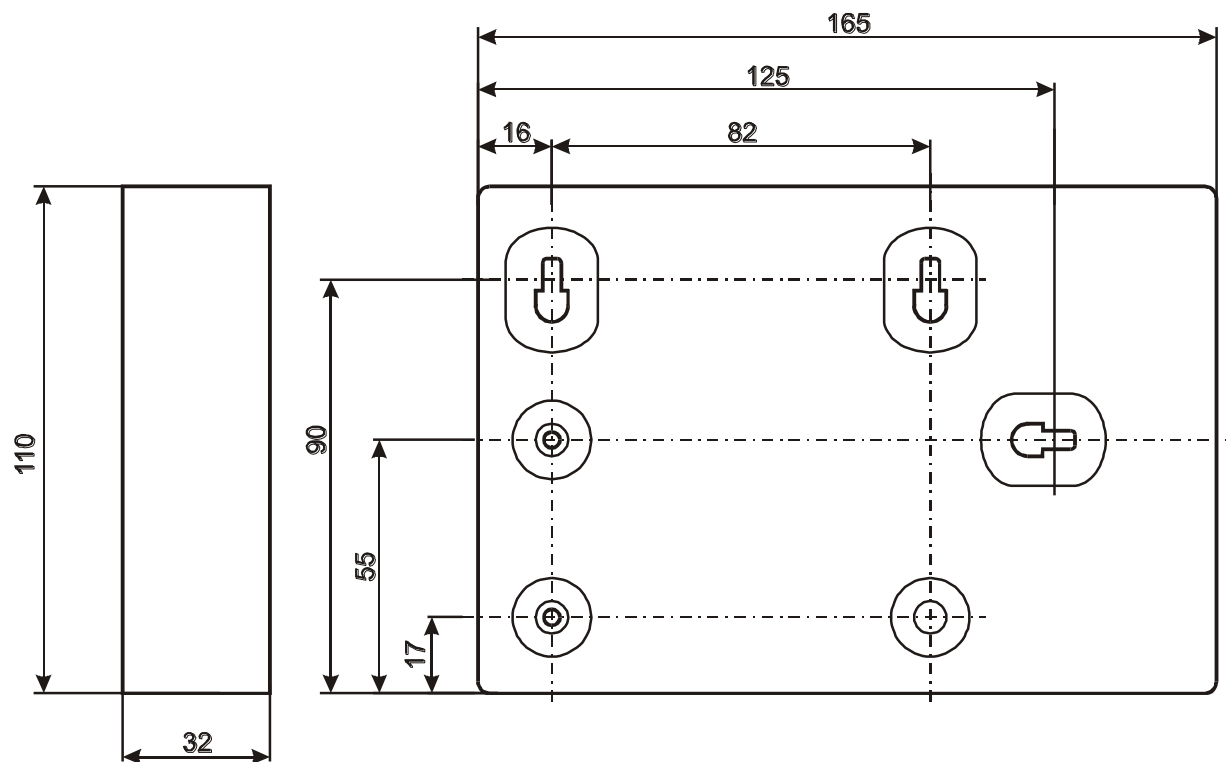
Рис. 2 Внешний вид, габаритные и присоединительные размеры (исполнение IP20)
