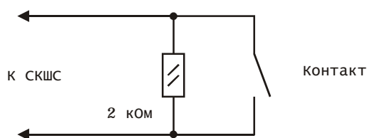
Рис. 3 Схема включения ШС с контролем обрыва
