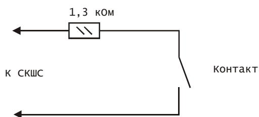
Рис. 4 Схема включения ШС с контролем КЗ
