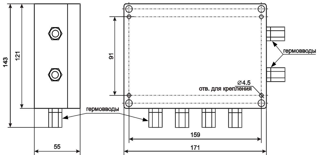
Рис. 6 Внешний вид, габаритные и присоединительные размеры (исполнение IP20)
