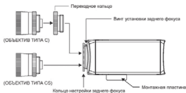
ВИД СБОКУ
