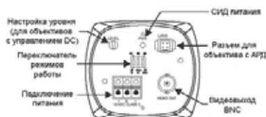
ВИД СЗАДИ (12 В пост. тока)
