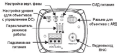
ВИД СЗАДИ (24 В пер. тока)
