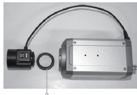
C-крепление объектива (необходимо переходное кольцо)
