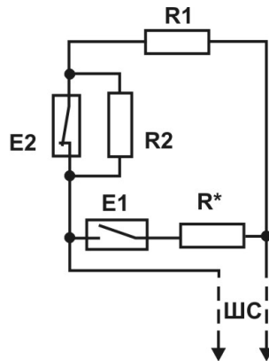
Рисунок 2. Схема подключения комбинированного пожарного шлейфа
