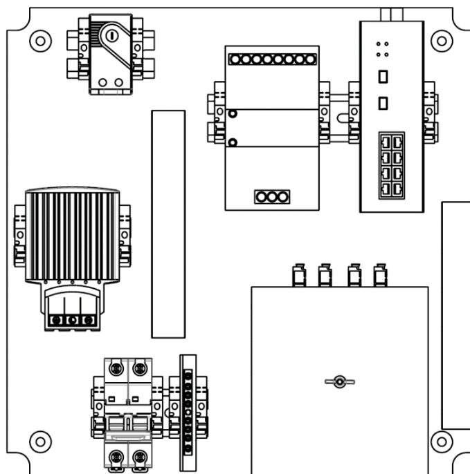
Рисунок 1 – Устройство шкафа
