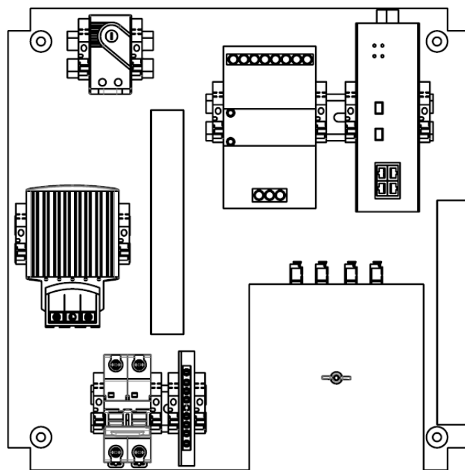
Рисунок 1 – Устройство шкафа
