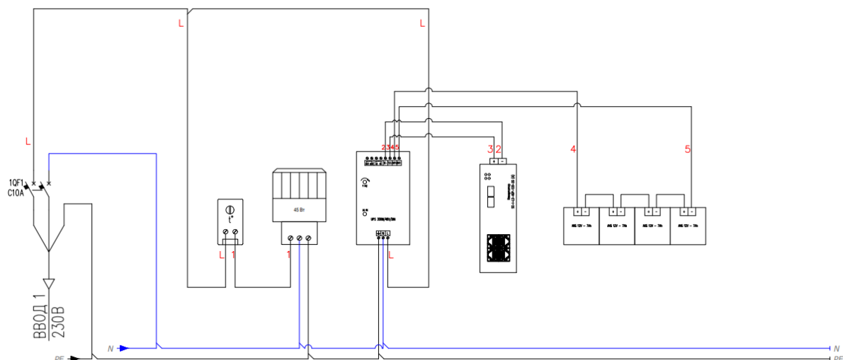
Рисунок 2 – Схема электрическая принципиальная
