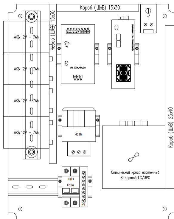
Рисунок 1 – Устройство шкафа
