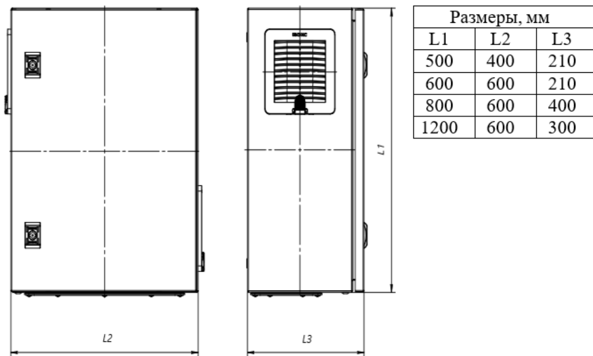
Рис. 1 – Габаритные размеры термощкафа
