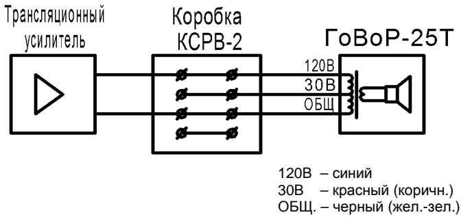
Рис. Б.1. Схема подключения ГоВоР-25Т.
