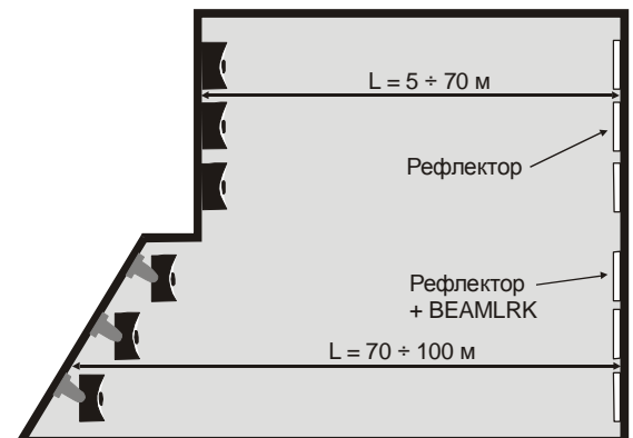
Рис. 13. Извещатели и рефлекторы крепятся на стену. При угле установки больше 10° относительно друг друга извещатели крепятся с помощью кронштейнов 6500-ММК, а рефлекторы 6500-LRK крепятся непосредственно на стену.
