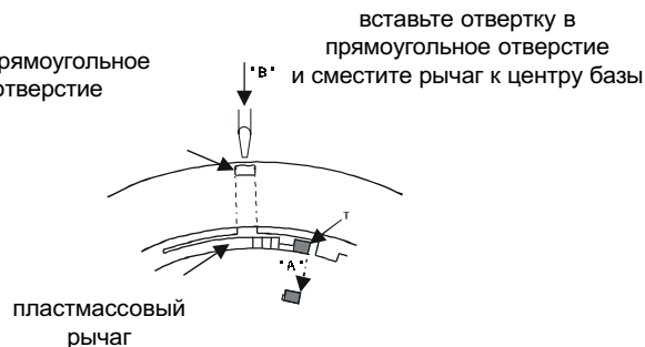
Рис. 5. Извлечение извещателя из базы после активизации защиты
