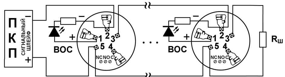
Рис. 3. Типовая 2-х проводная схема подключения базовых оснований B424RL к ПКП
