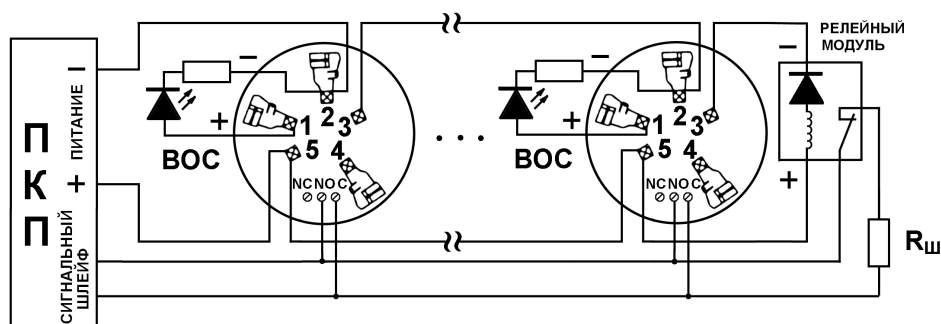
Рис. 2. Типовая 4-х проводная схема подключения базовых оснований B424RL к ПКП (контакты релейного модуля показаны при включенном напряжении питания)
