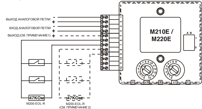
РИС.3. МОНТАЖ ШЛЕЙФОВ M210E С ОДНИМ КАНАЛОМ КОНТРОЛЯ И M220E С ДВУМЯ КАНАЛАМИ КОНТРОЛЯ
