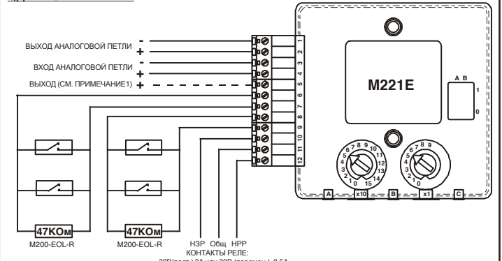
РИС.3. МОНТАЖ ШЛЕЙФОВ M221E С ДВУМЯ КАНАЛАМИ КОНТРОЛЯ И ОДНИМ УПРАВЛЕНИЯ
