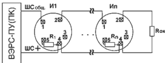
Рис. 3. Подключение извещателей серии ЕСО1000 в режиме распознавания срабатывания двух извещателей в шлейфе
