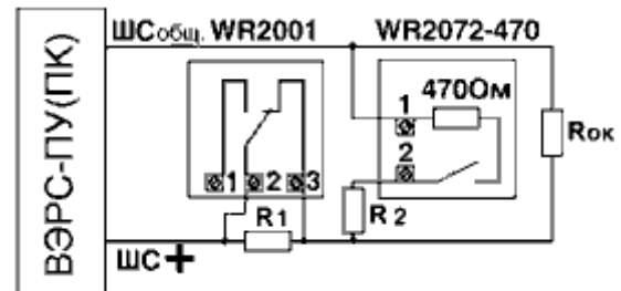
R1 - резистор 5,4 кОм ± 5%; R2 - резистор 1,3 кОм ± 5%; Rок - оконечный резистор шлейфа - 7,5 кОм±5%
