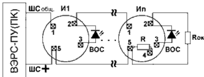
И1,..., Ип - n извещателей серии ЕСО1000 с базами Е1000В и Е1000R R - резистор в базе Е1000R (не используется) Rок - резистор 7,5 - 10 кОм оконечный элемент шлейфа, выбирается в зависимости от количества извещателей в шлейфе
