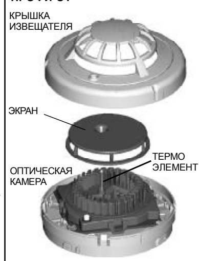
Рис. 3. Комбинированный извещатель ИП212/101-4-A1R ПРОФИ-ОТ
