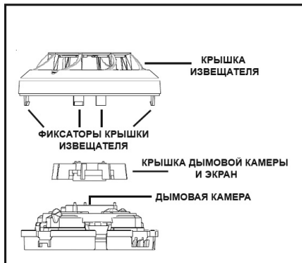
Рис.2: Обслуживание извещателя
