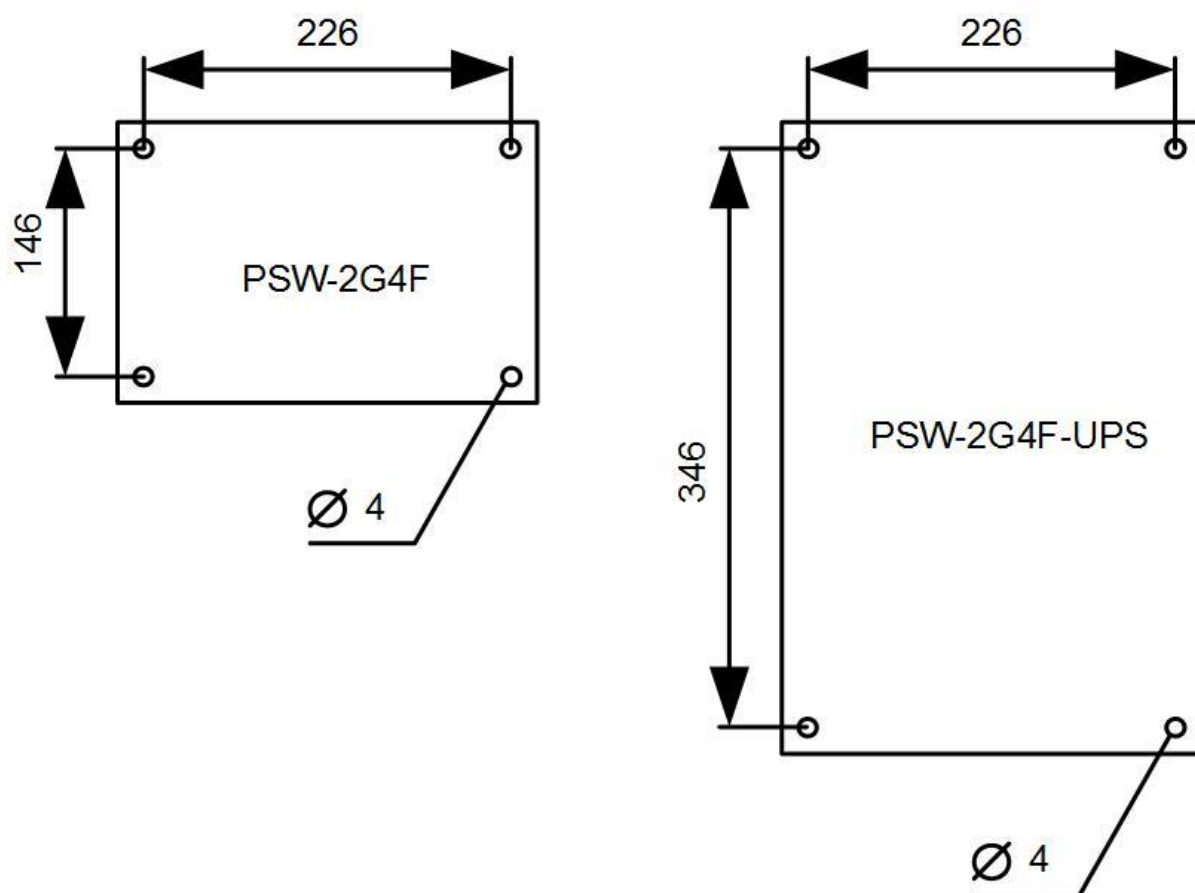
Рис. 6.1.1. Разметка крепления
