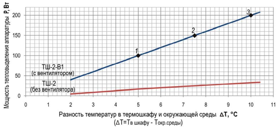
График 1 Зависимость мощности тепловыделения устанавливаемой в термощкафу аппаратуры от разности температур в термощкафу и окружающей среды
