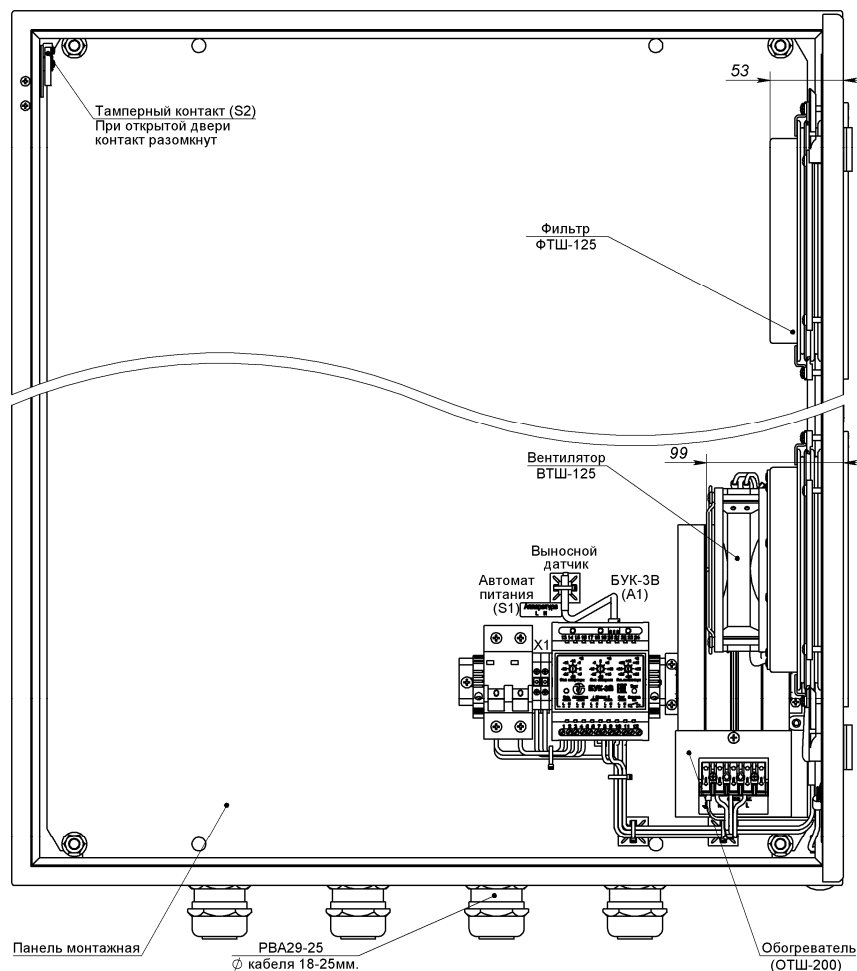
Рис. 1. Устройство термощафа (дверь открыта на 90°)
