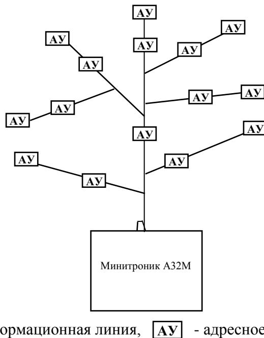
Рис. 6. Архитектура лучевой информационной линии с ответвлениями.
