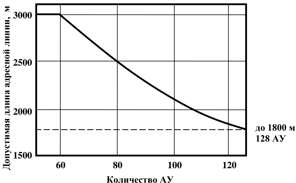
Рис. 8. Допустимая длина линейной части адресной линии в зависимости от количества АУ (допустимая длина определяется как максимальное удаление АУ от любой из клемм прибора).
