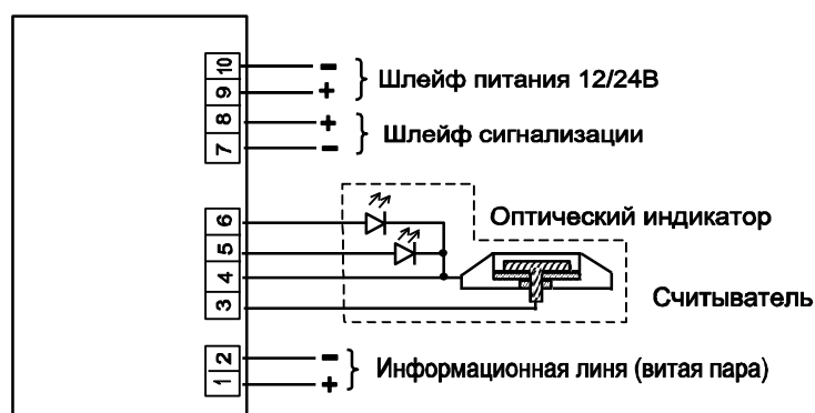
Рис. 2. Схема подключения модуля адресации.
