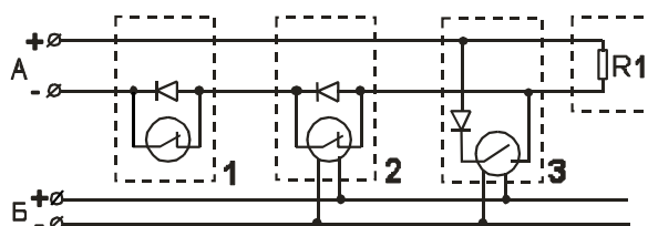
Рис. 2. Схема подключения модуля адресации.
