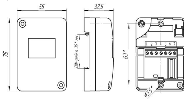
Рис.1. Габаритные и установочные размеры модуля.
