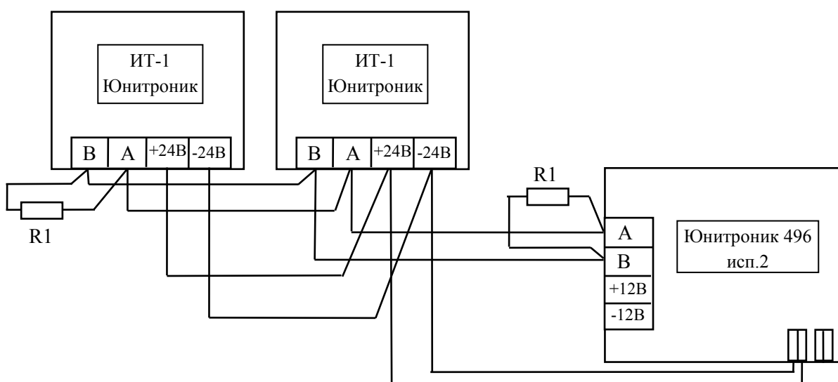
Рис. 11. Схема подключения информационного табло к прибору. R1= 100 Ом±5%.
