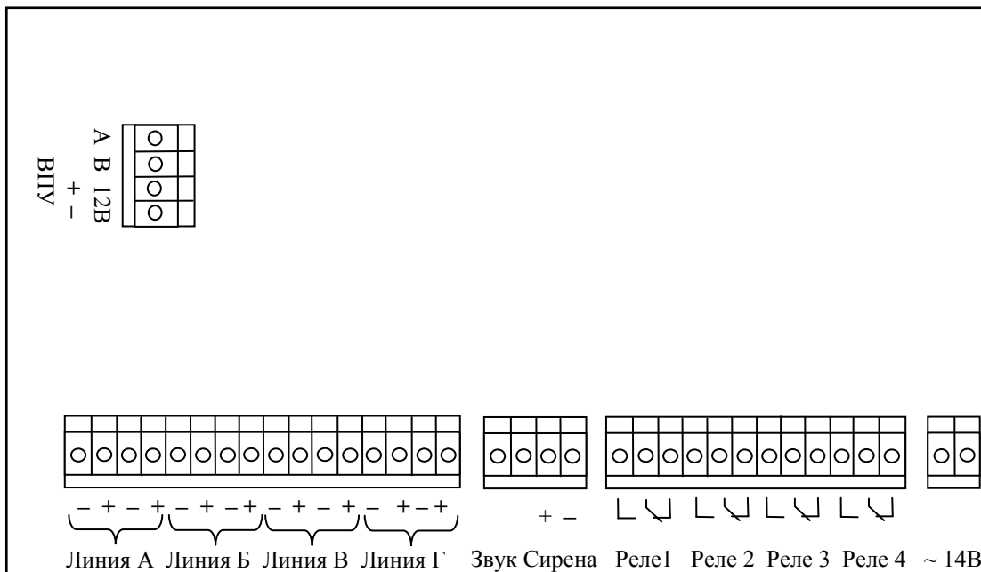
Рис. 8. Расположение клемм подключения на системной плате АПКП.
