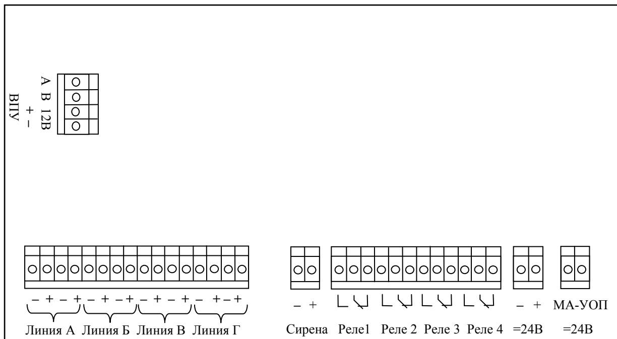
Рис. 10. Расположение клемм подключения на системной плате АПКП «Юнитроник 496 исп.2».
