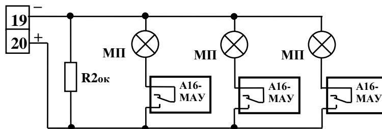
Рис.4. Схема подключения модулей пожаротушения ("МП") с контролем исправности цепи каждого модуля. R_{2ок} = 10 \text{ кОм} ( 0,25Вт , \pm 5\% ). При количестве модулей А16-МАУ более 4-х резистор R_{2ок} допускается не устанавливать.
