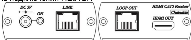
Рис.7 Панель подключения HE01SLR
