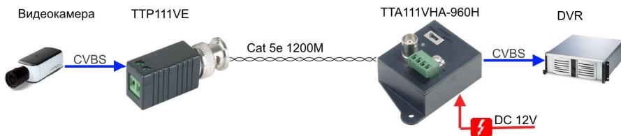
Рис.4 Схема подключения TTP111VE и TTA111VHA-960H.
