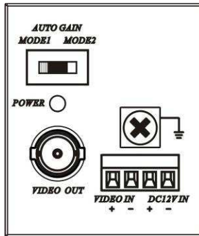
Рис.2 Разъёмы ТТА111VHA-960Н.
