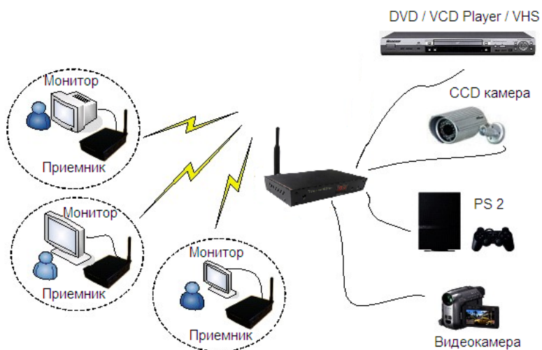
Рис.3 Схема подключения (один передатчик – несколько приемников)
