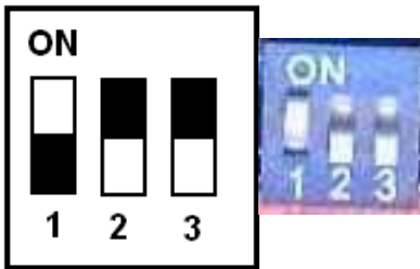
Рис.11 Внешний вид DIP-переключателей.
