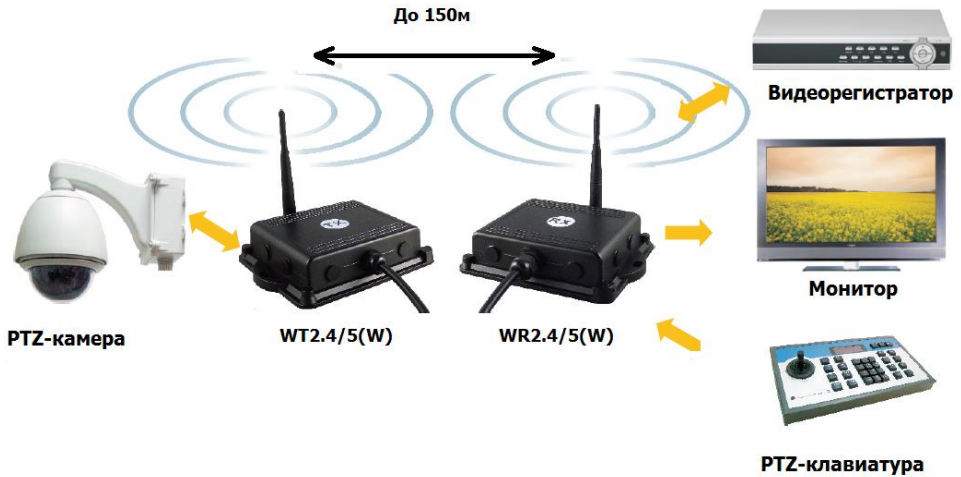
Рис.3 Схема подключения передатчика WT2.4/5(W) и приёмника WR2.4/5(W).
