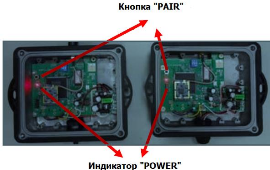
Рис.7 Сопряжение передатчика и приёмника.
