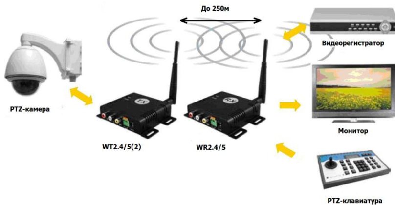
Рис.4 Схема подключения передатчика WT2.4/5(2) и приёмника WR2.4/5.
