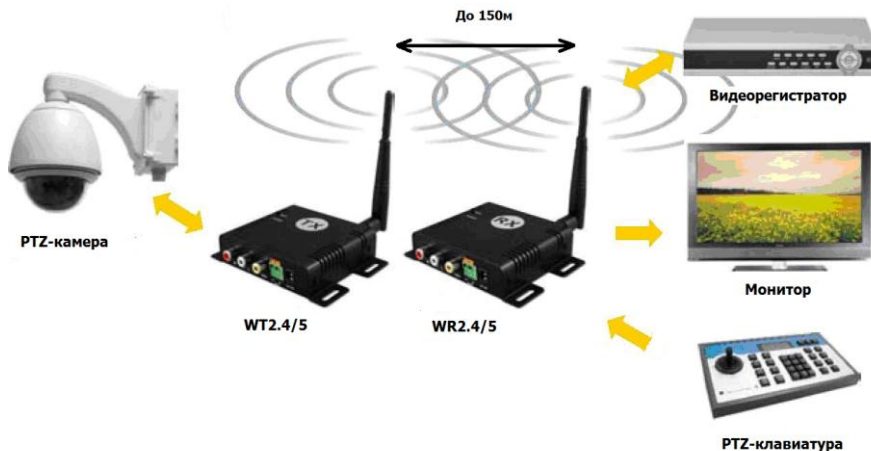
Рис.3 Схема подключения передатчика WT2.4/5 и приёмника WR2.4/5.
