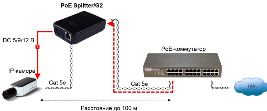
Рис. 4. Схема подключения сплиттера PoE Splitter/G2
