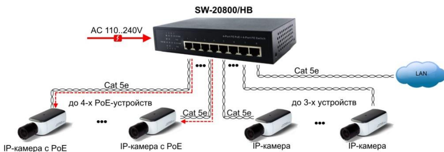
Рис. 3 Схема подключения коммутатора SW-20800/HB
