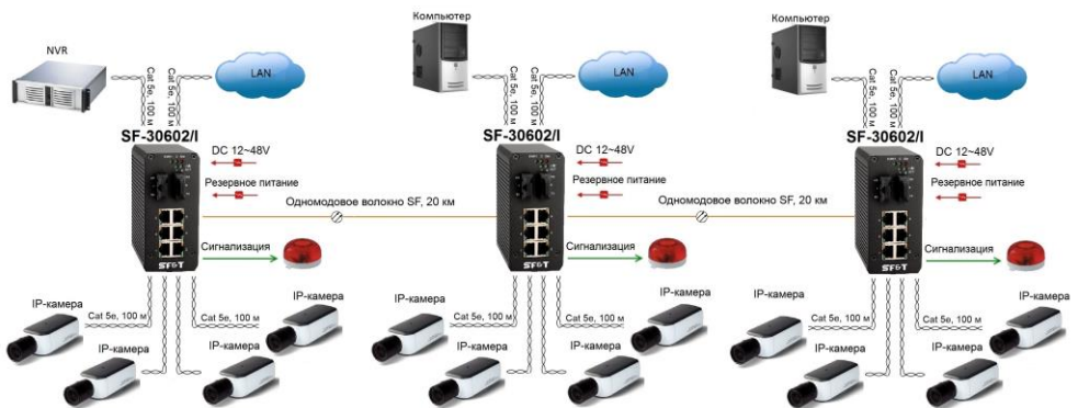
Рис.6 Схема подключения трех коммутаторов SF-30602/I
