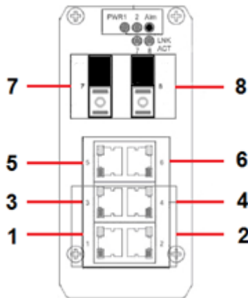
Рис.3 Порты коммутатора SF-30602/I
