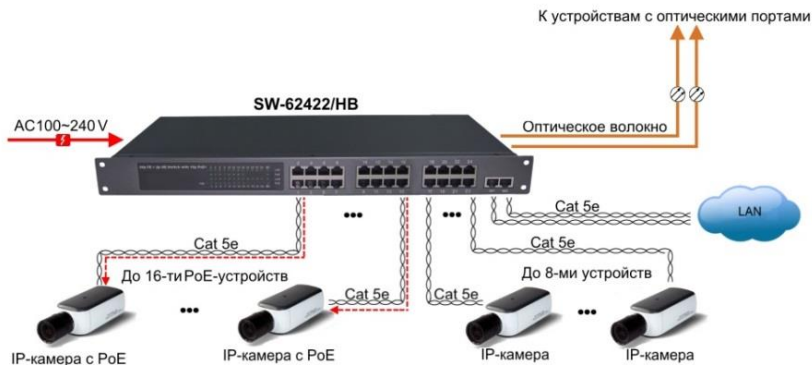
Рис. 4 Схема подключения коммутатора SW-62422/HB Технические характеристики
