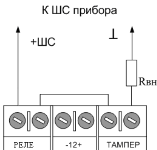
Рисунок 1 – Схема подключения извещателя в шлейф сигнализации
