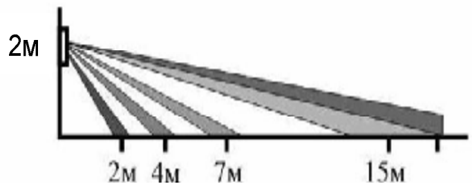
Рис. 2. Диаграмма элементарных чувствительных зон извещателя
