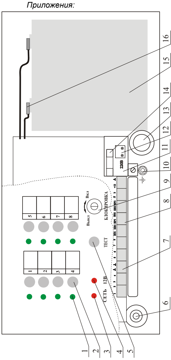
Рис. 1. Внешний вид и устройство приборов «ВЭРС-ПК2», «ПК4», «ПК8»
