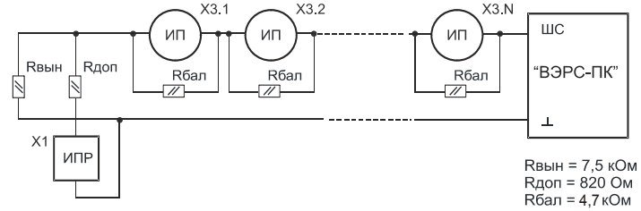
Рис. 9. Схемы включения ШС с несколькими тепловыми извещателями (типа ИП-105) и сработкой по двум извещателям (с перезапросом)
