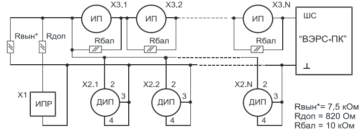
Рис. 10. Комбинированная схема включения ШС со сработкой по одному извещателю (с перезапросом)
