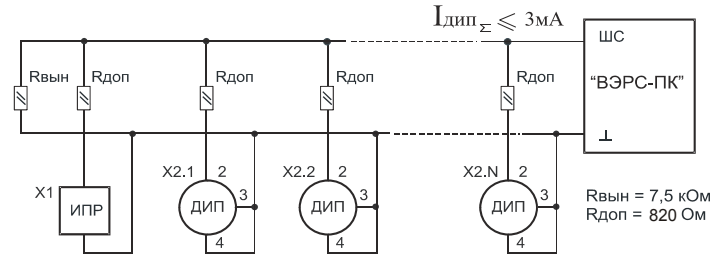
Рис. 8. Схемы включения ШС с несколькими дымовыми извещателями (типа ИП212) и сработкой по двум извещателям (с перезапросом)
