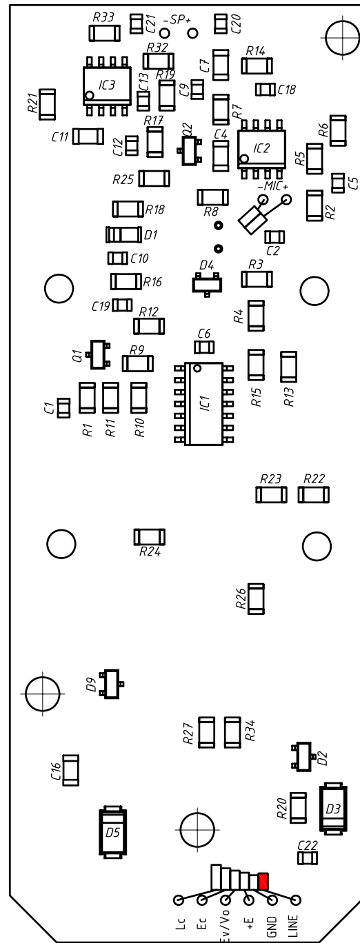
Плата БВД-403А Сборочный чертеж
