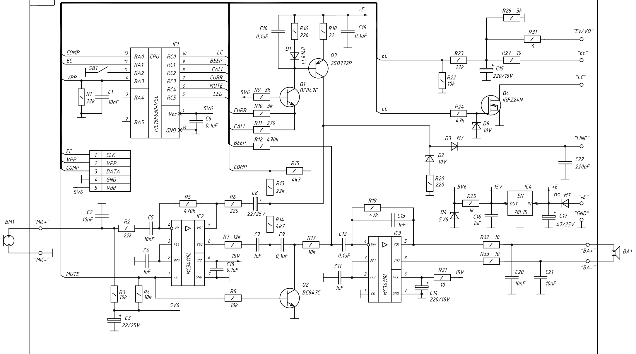
Блок вызова БВД-403А Схема электрическая принципиальная
