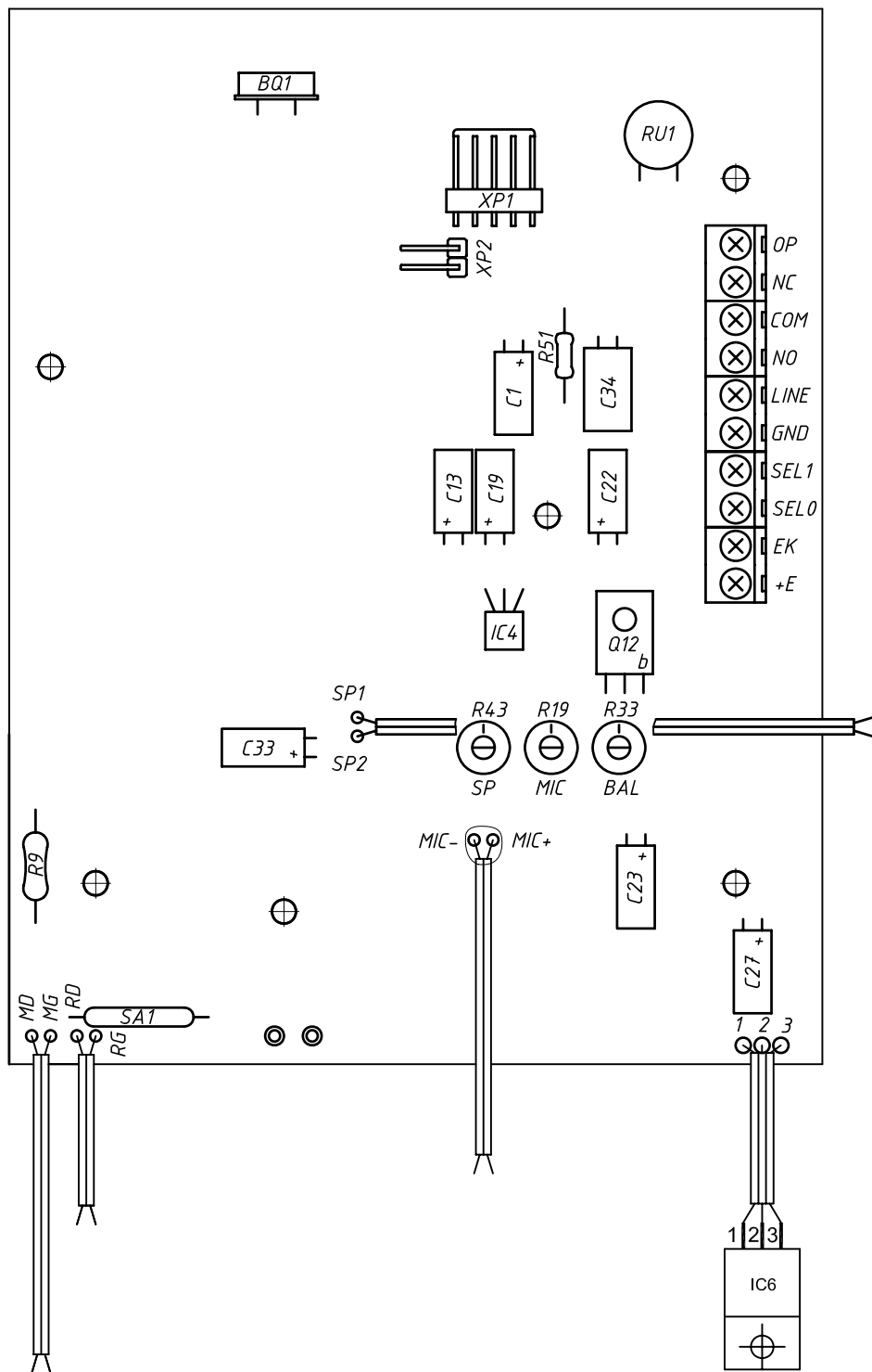
Плата БВД-М200 Сборочный чертёж
