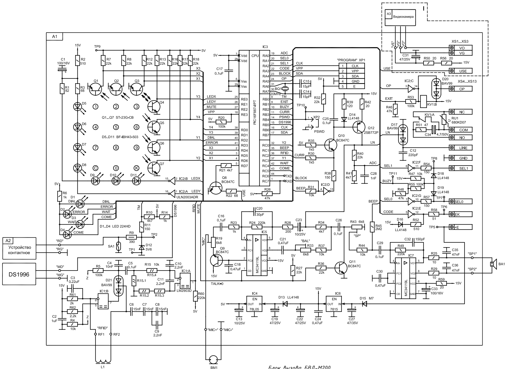
Блок вызова БВД-М20 Схема электрическая принципиальная
