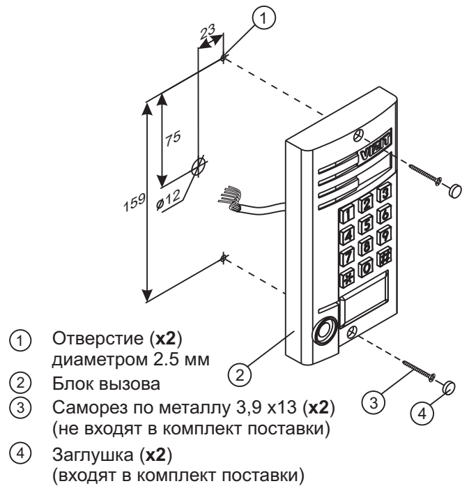
Рисунок 3 - Установка блока на неподвижную часть металлической двери
