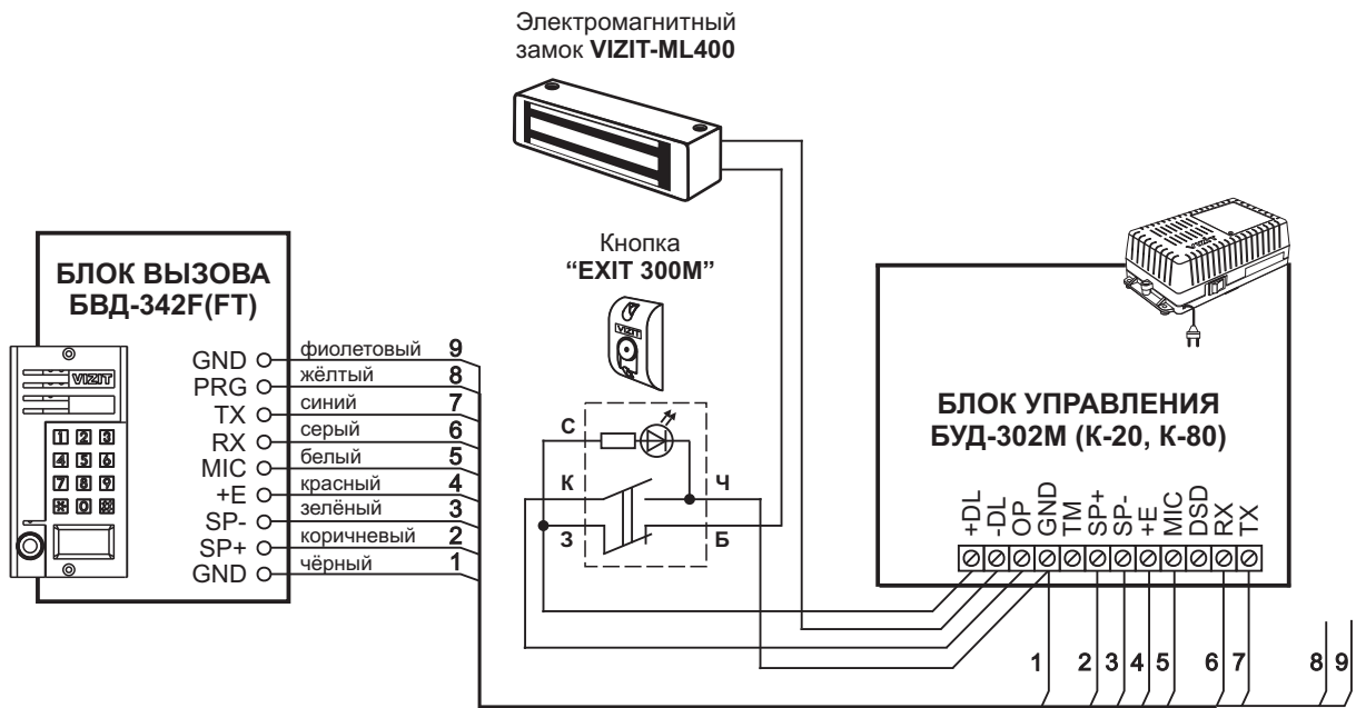
Рисунок 4 - Схема соединений блока вызова БВД-342F(FT) с блоком управления БУД-302М (К-20, К-80) , электромагнитным замком VIZIT-ML400 и кнопкой "EXIT 300М"
