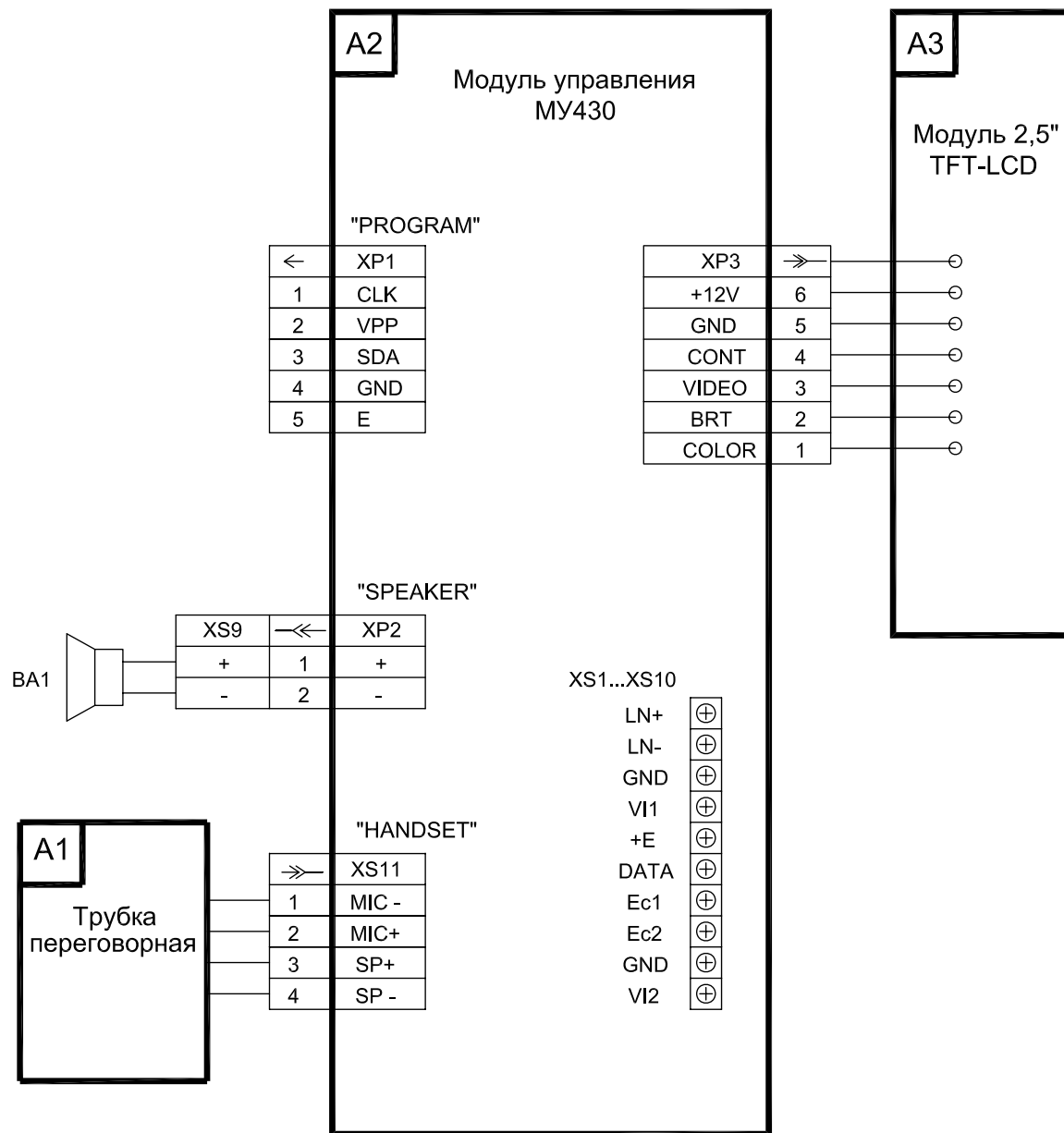
Монитор VIZIT-M430C Схема соединений
