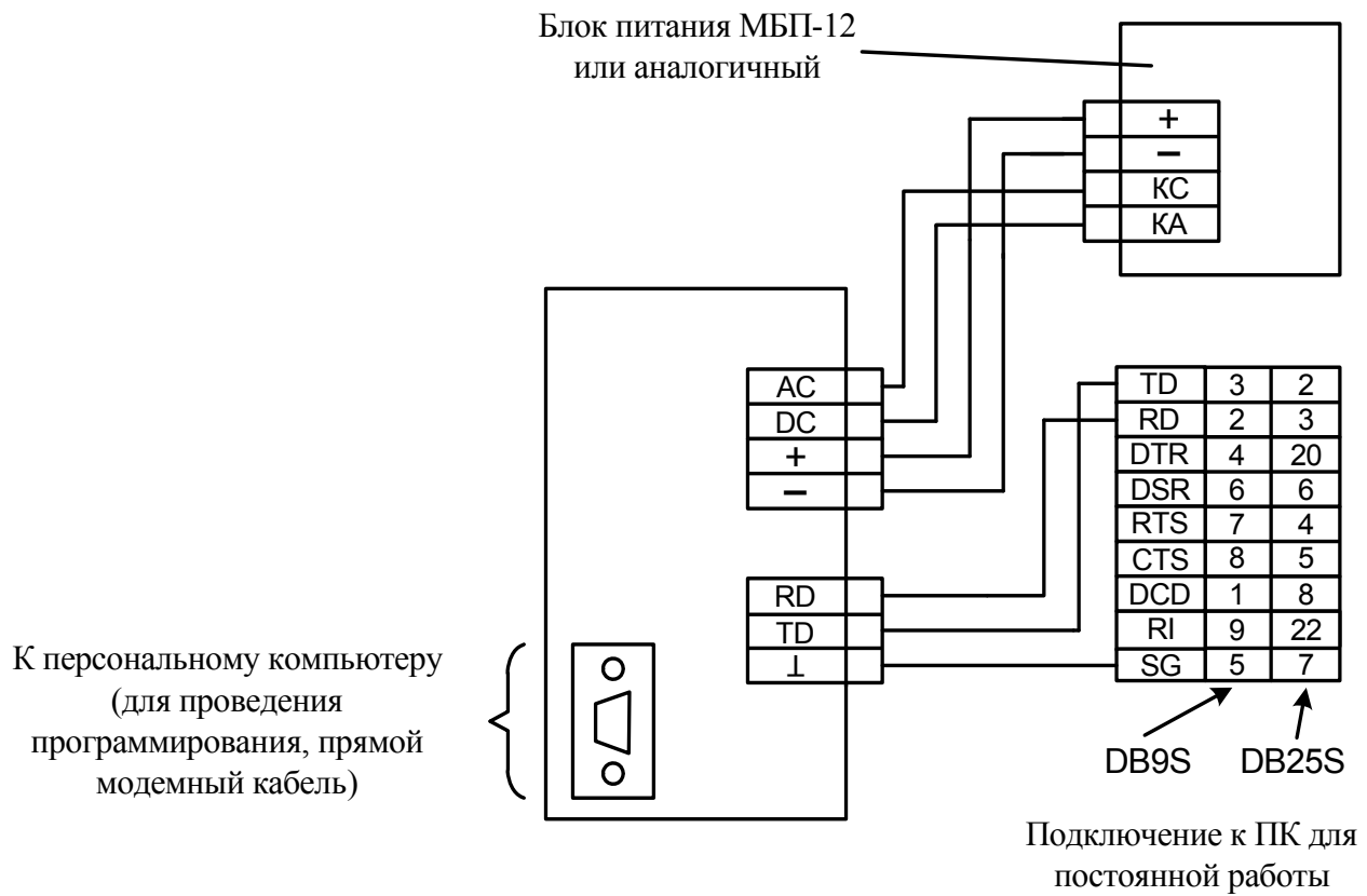
Рисунок В.6 – Схема внешних подключений РРОП-М
