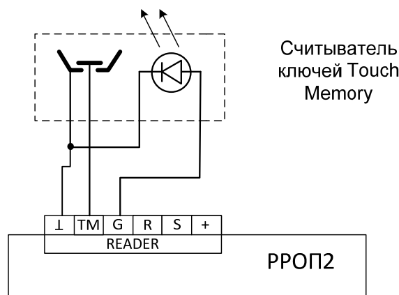
б) Подключение считывателя ключей Touch Memory
