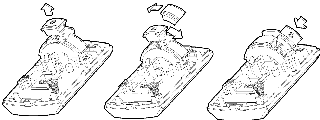
Рисунок Б.2 – Позиционирование микрофона
