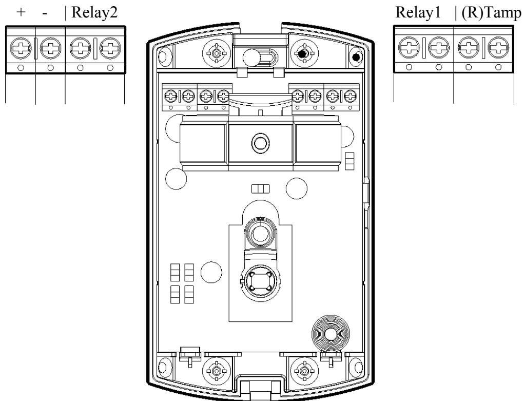
Рисунок Б.1 – Внешний вид извещателя
