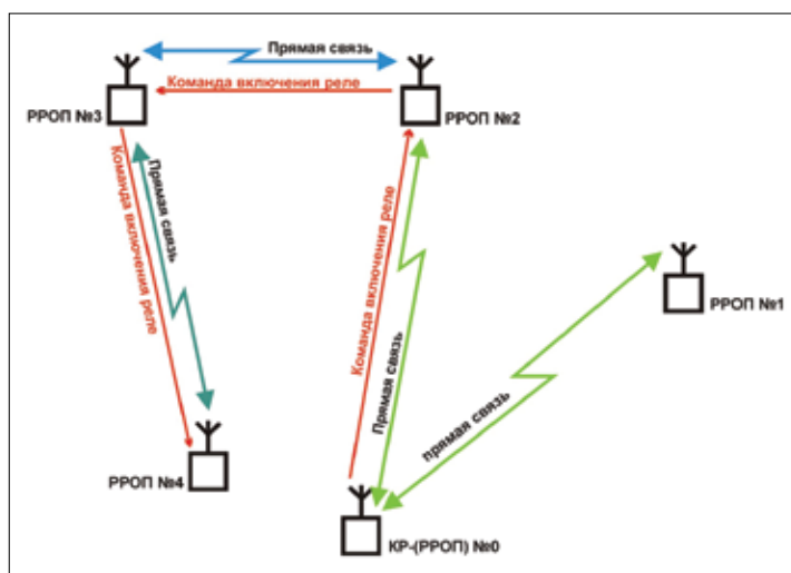
Рис.3 Радиосистема СТРЕЛЕЦ® со статической маршрутизацией
