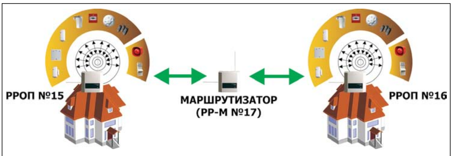
Рис. 6 Дополнительные 16 радиорасширителей-маршрутизаторов (РР-М)
