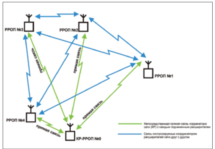
Рис. 5 Радиосистема СТРЕЛЕЦ® с динамической маршрутизацией
