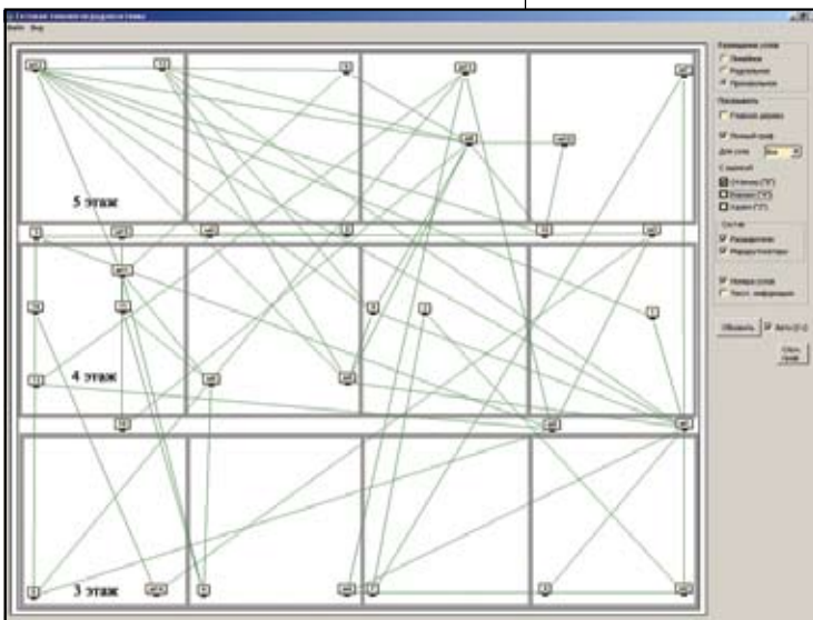
Рис. 9 Полный граф радиосистемы СТРЕЛЕЦ® на графическом плане
