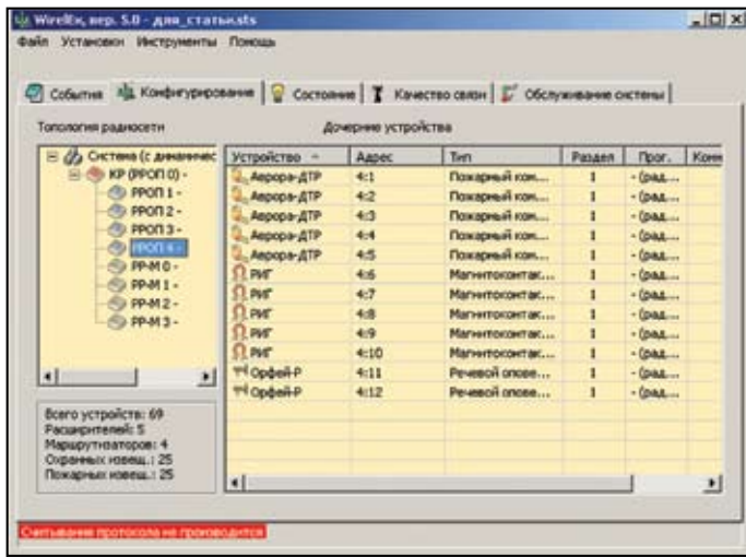
Рис. 4. Конфигурация радиосистемы СТРЕЛЕЦ® с динамической маршрутизацией
