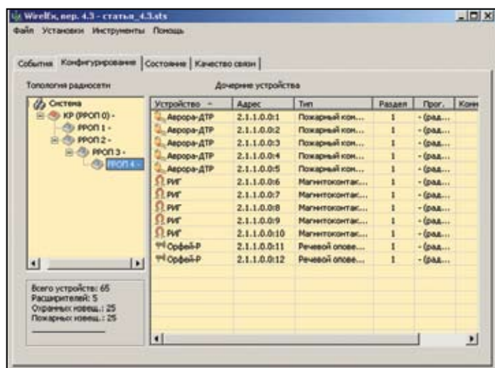
Рис.2. Конфигурация радиосистемы СТРЕЛЕЦ® со статической маршрутизацией
