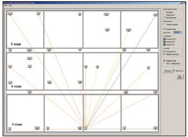
Рис. 11 Полный граф радиосистемы СТРЕЛЕЦ® для узла №1
